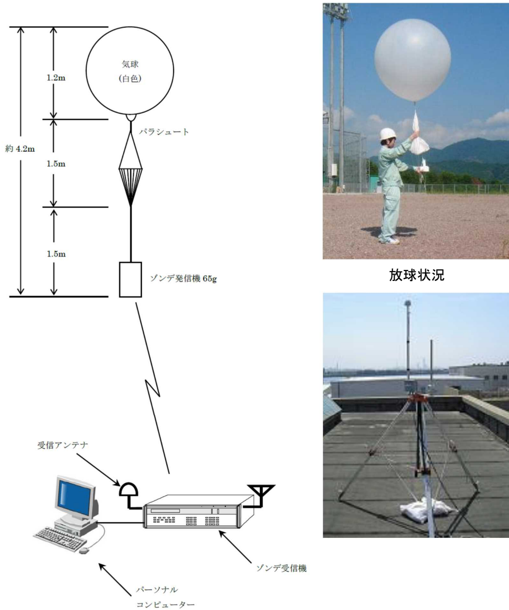
図 2 GPS ゾンデによる上層気象観測概略図
